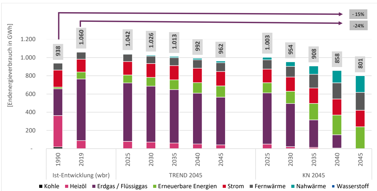
Abbildung 32 Entwicklung Endenergieverbrauch Haushalte in den Szenarien
