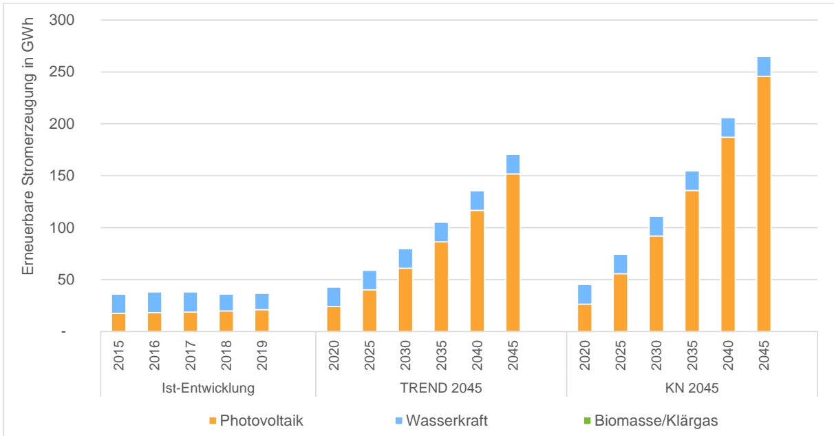
Abbildung 43 Entwicklung der lokalen Stromerzeugung aus erneuerbaren Energien bis zum Jahr 2045 Quelle: Berechnung und Darstellung IE Leipzig Anmerkung: Stromerzeugung aus KWK-Prozessen auf Basis erneuerbarer Energien (vgl. Kapitel Wärmeerzeugung) wurde in der Darstellung nicht berücksichtigt
