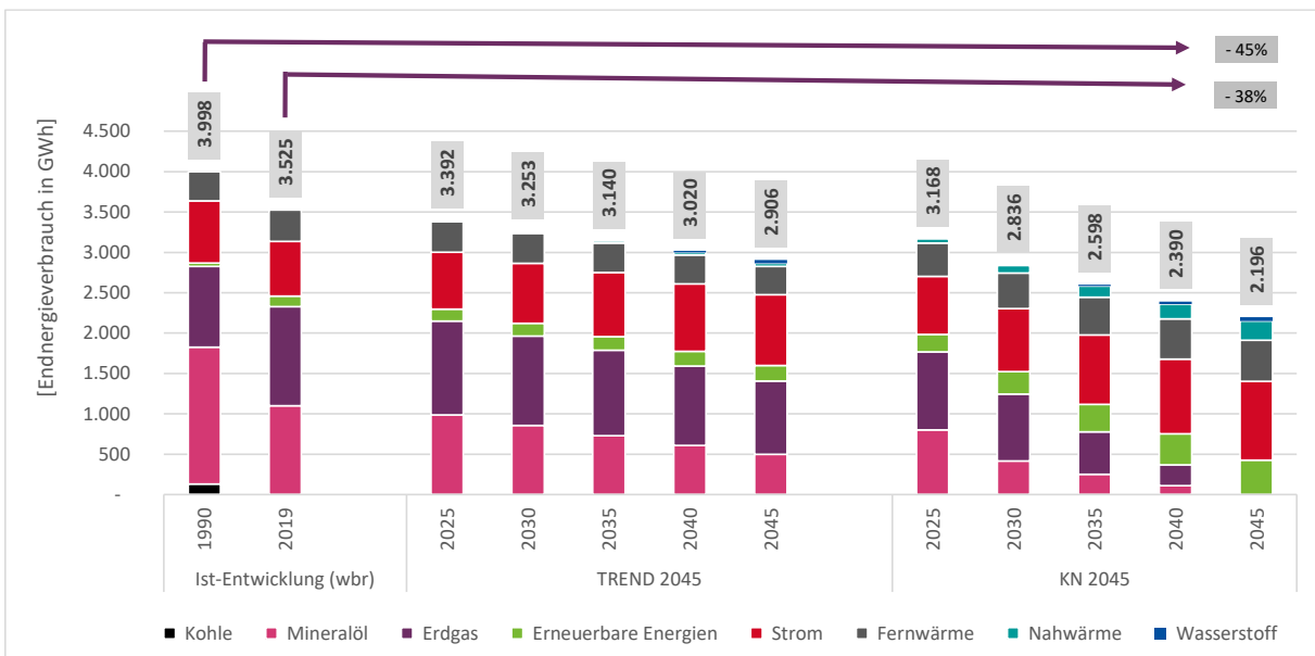
Abbildung 45 Entwicklung Endenergieverbrauch nach Energieträgern in den Szenarien Quelle: Berechnung und Darstellung IE Leipzig
