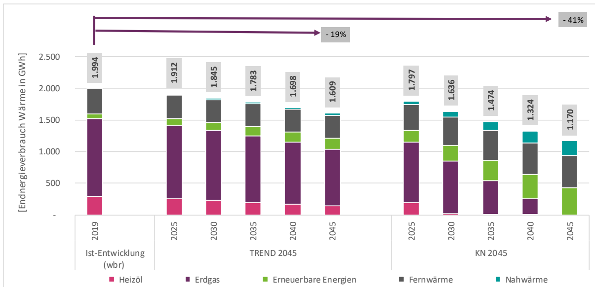
Abbildung 41 Entwicklung der Wärmeversorgung bis zum Jahr 2045 Quelle: Berechnung und Darstellung IE Leipzig
