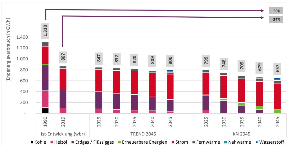
Abbildung 34 Entwicklung Endenergieverbrauch Industrie in den Szenarien
