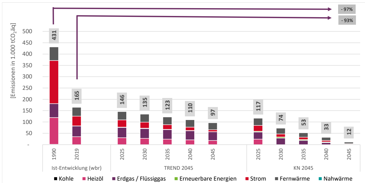
Abbildung 37 Entwicklung Emissionen GHD in den Szenarien Quelle: Darstellung und Berechnung IE Leipzig
