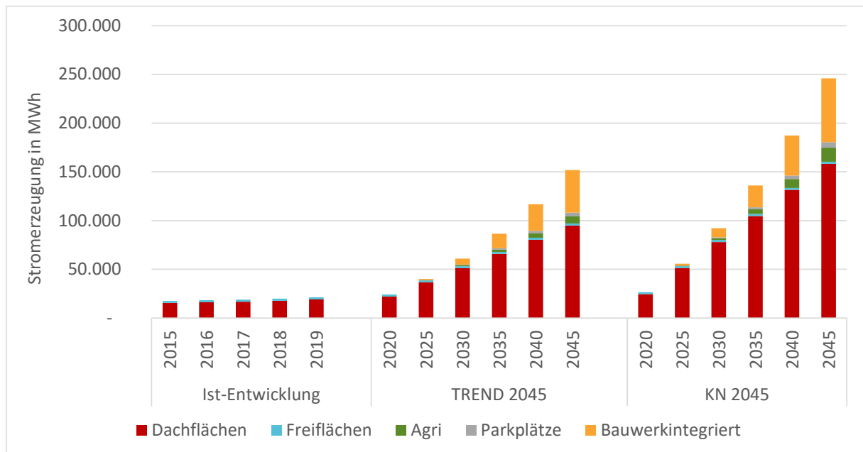
Abbildung 42 Entwicklung der Stromerzeugung aus Photovoltaikanlagen bis zum Jahr 2045
