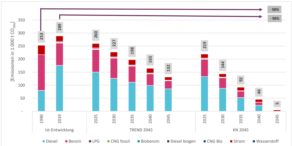
Abbildung 39 Entwicklung Emissionen Verkehr in den Szenarien
