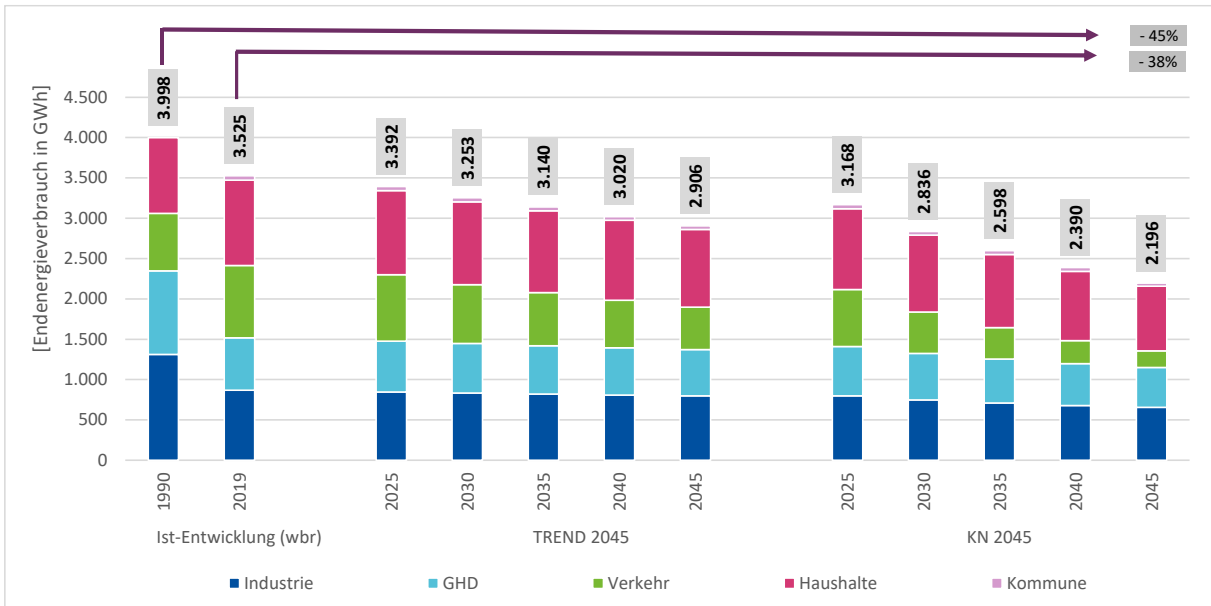
Abbildung 44 Entwicklung Endenergieverbrauch nach Sektoren in den Szenarien Quelle: Berechnung und Darstellung IE Leipzig
