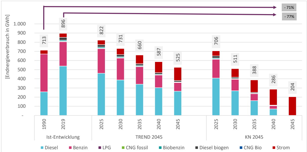
Abbildung 38 Entwicklung Endenergieverbrauch Verkehr in den Szenarien
