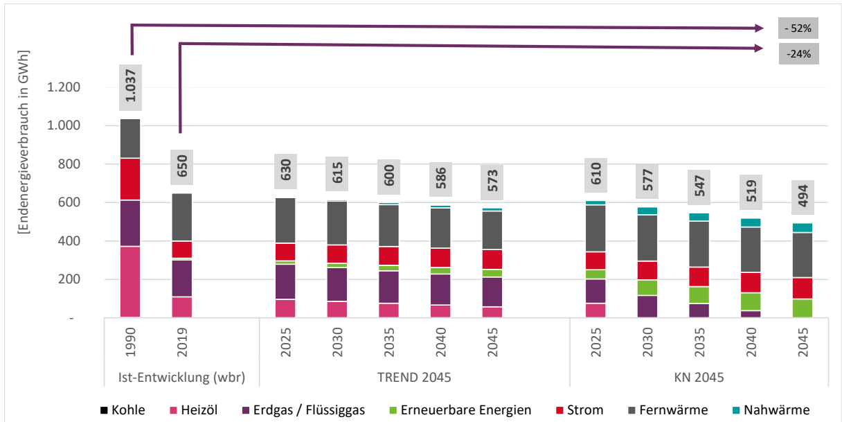
Abbildung 35 Entwicklung Endenergieverbrauch GHD in den Szenarien Quelle: Darstellung und Berechnung IE Leipzig
