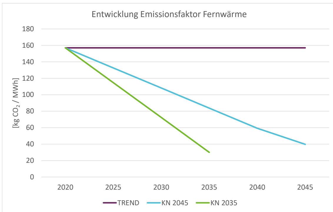
Abbildung 40: Annahmen zur Entwicklung des Emissionsfaktors der Fernwärme Quelle: IE Leipzig 2021
