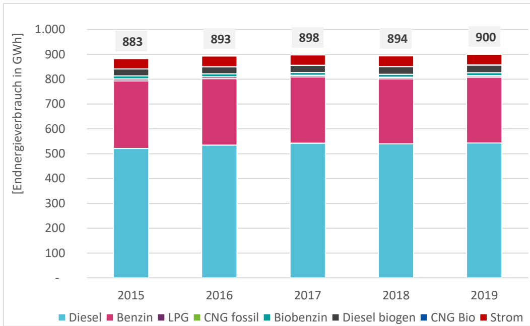
Abbildung 22 Endenergieverbrauch Verkehr (nicht wbr) nach Energieträgern 2015 bis 2019 Quelle: Darstellung IE Leipzig
