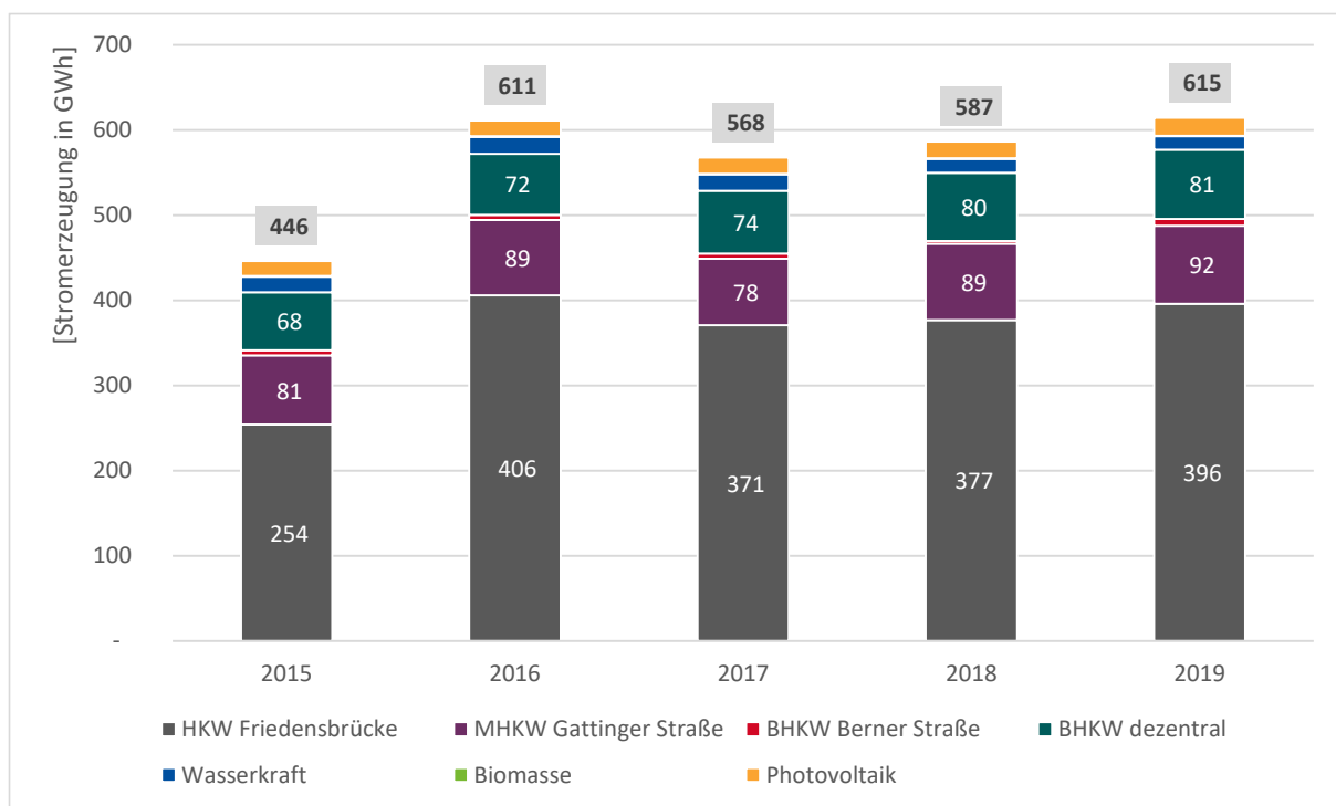
Abbildung 24 Netzeinspeisung Strom nach Energieträgern 2015 bis 2019
