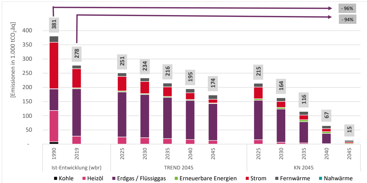
Abbildung 33 Entwicklung Emissionen Haushalte in den Szenarien Quelle: Darstellung und Berechnung IE Leipzig
